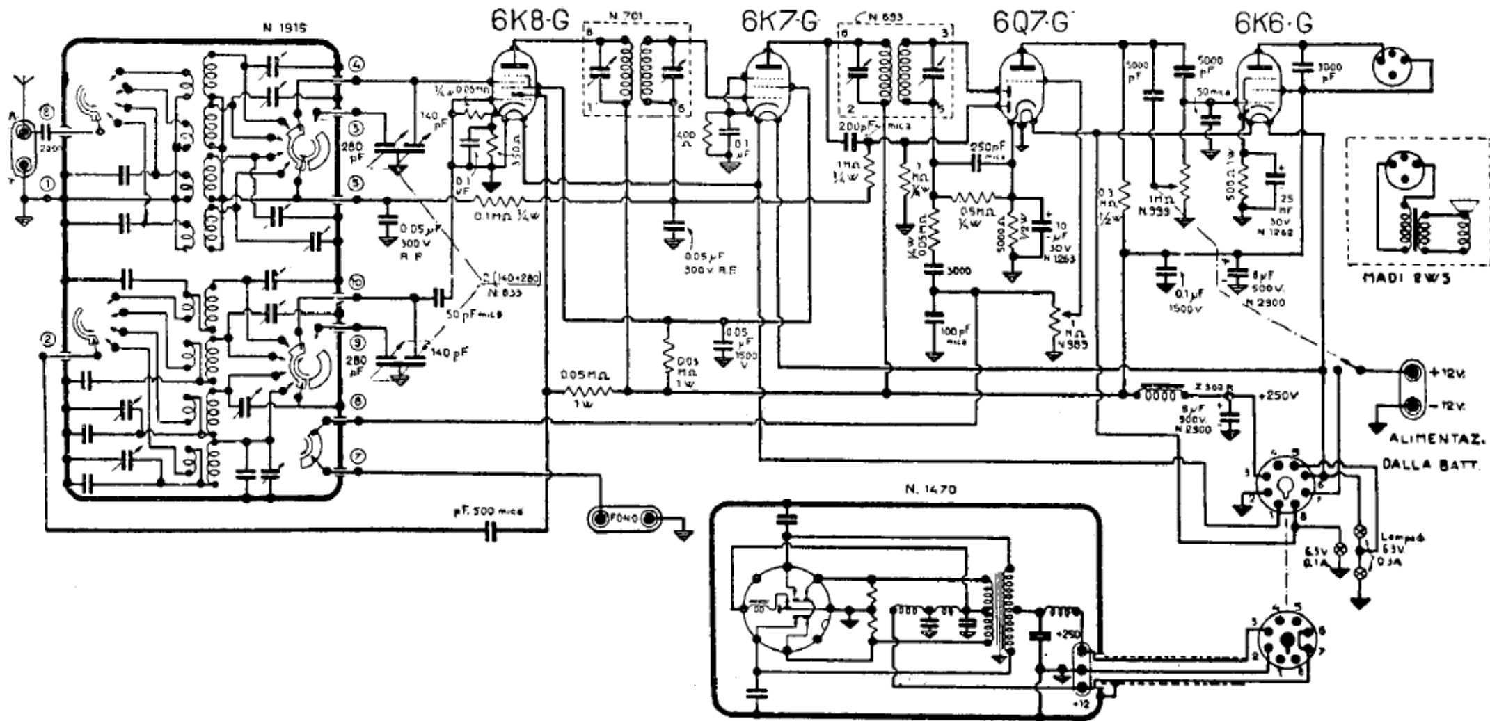
S. A. GELOSO. — Mod. G. 49. — Alimentazione da batteria d'accumulatori 12 V. con survoltore 1470. — Media frequenza: 467 kHz. — Produzione 1940-1941.
